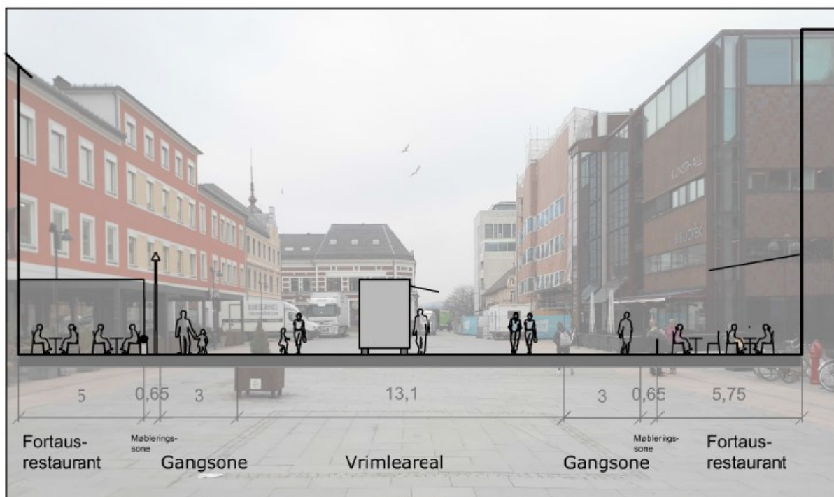
Figur 2 Snitt av nedre del av Torvet slik det nå er utformet
