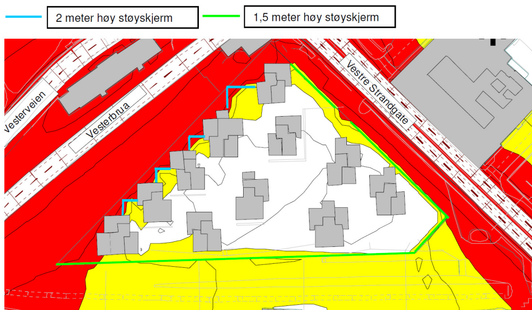
Figur 8 Beregnet lydtryknivå L_{den} fra tog og vei, beregningshøyde 1,5 meter over terreng (i dBA, dB re. 20µPa). Med støyskjermer.
