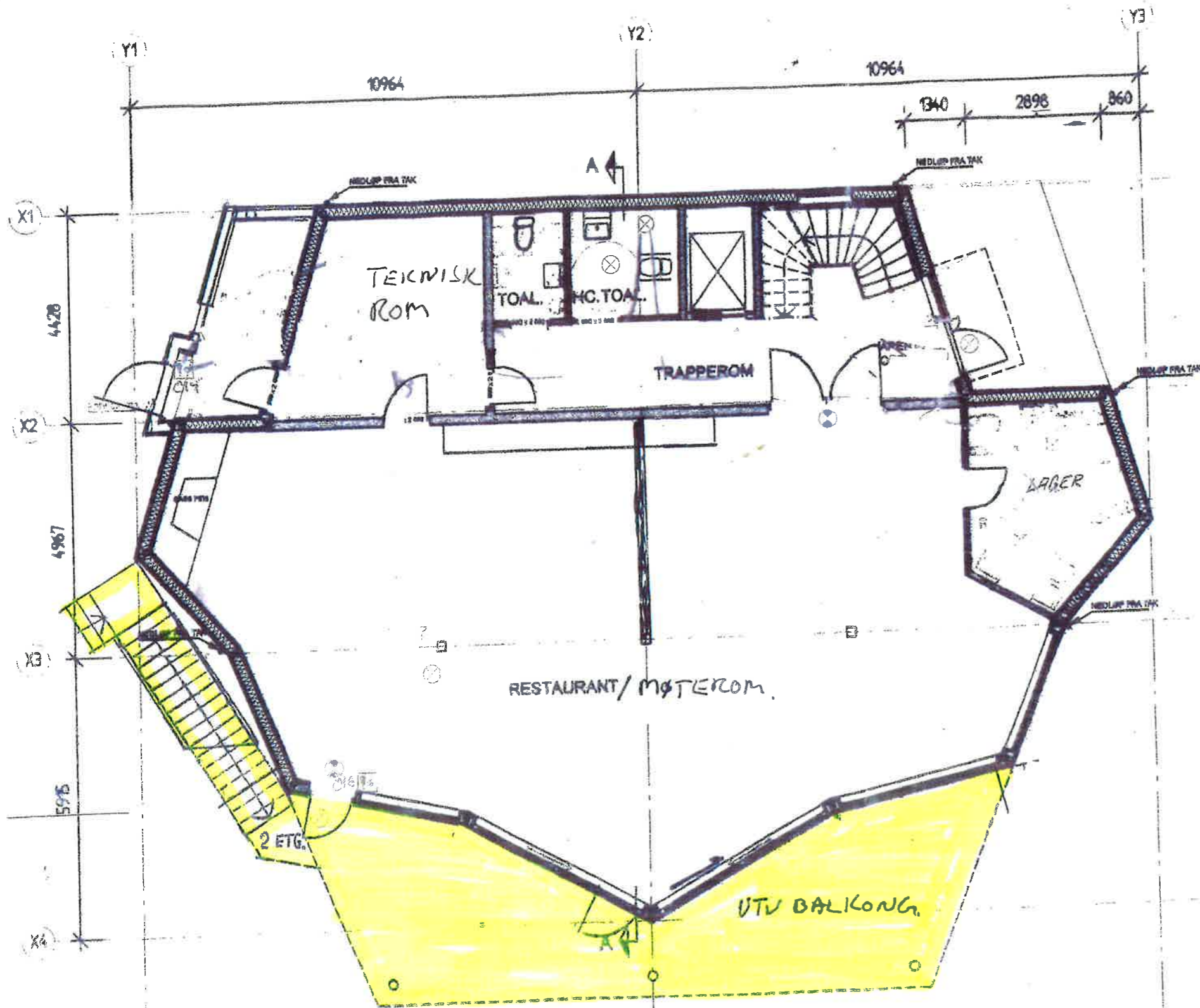
PLAN 2 ETASJE
